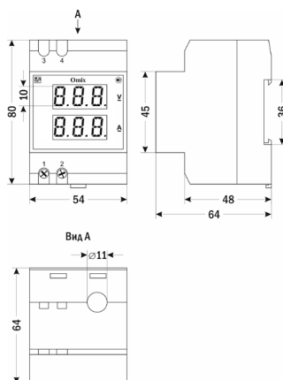
Рис. 2 – Размеры прибора
